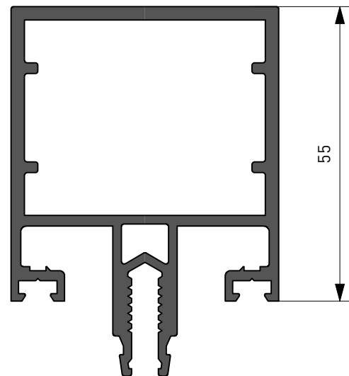
Peso 1.752 kg /ml. Ixx = 26 cm 4
