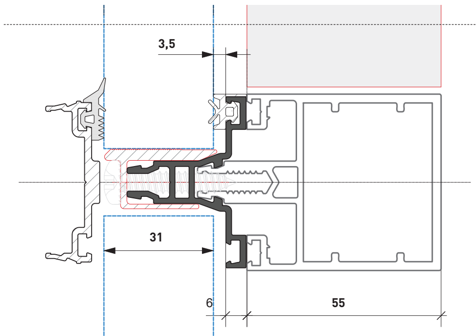
Sezione TRAVERSO
