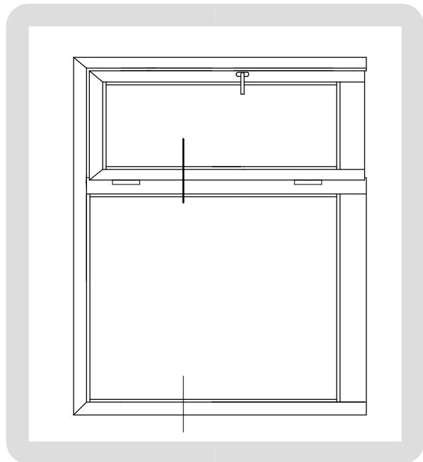
PORTA A 1 ANTA CON FISSO LATERALE
