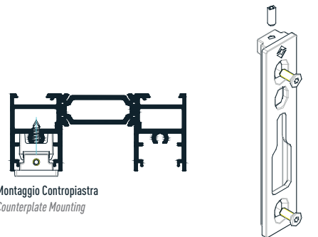
Installazione su Profilo Installation on Profile
