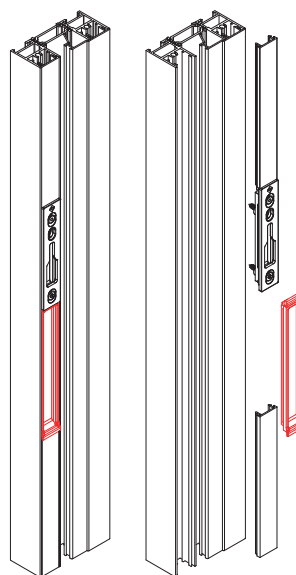
Aggiungere Cover ASX.08.80 Add covers ASX.08.80
