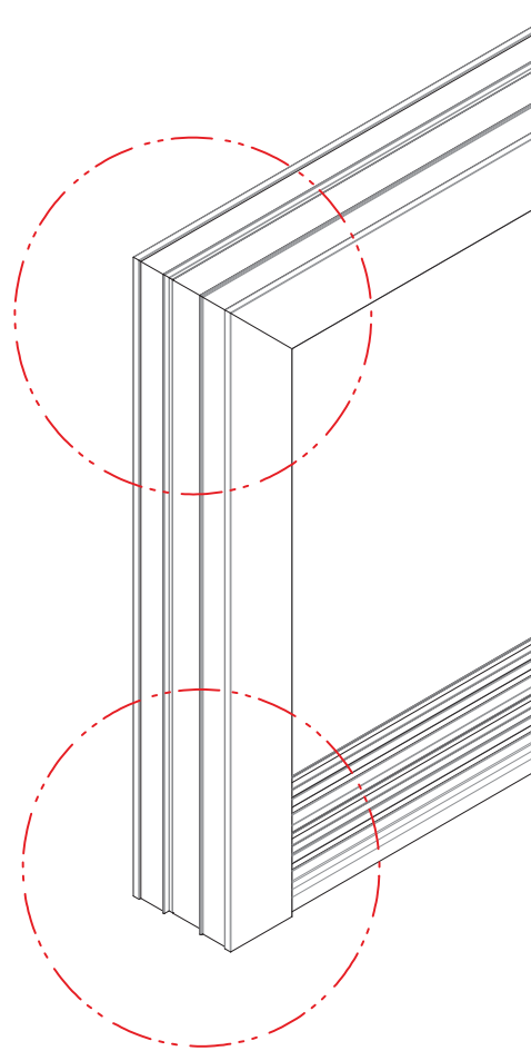
Asola e foro per squadretta (AWX 16.SQ) su profilo SX12.153 Slot and corner joint hole on profiles SX12.153
