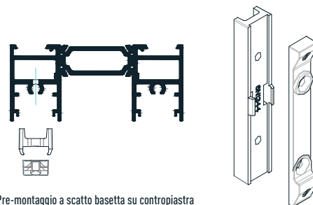
Pre-montaggio a scatto basetta su contropiastra Pre-mounted snap-on baseplate to counterplate
