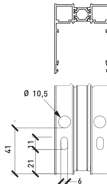
Asola e foro per squadretta (AWX 16.SQ) su profilo SX12.153 Slot and corner joint hole on profiles SX12.153
