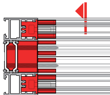
Sezione Orizzontale Horizontale Section
