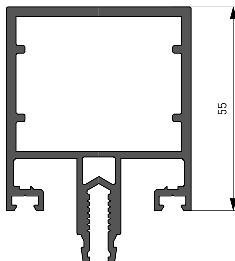
R6200 Peso 1.752 kg /ml. Ixx = 26 cm 4
