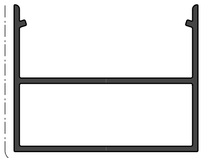
R 6229 Peso 0.673 kg./ml. -- mm. 550.0
