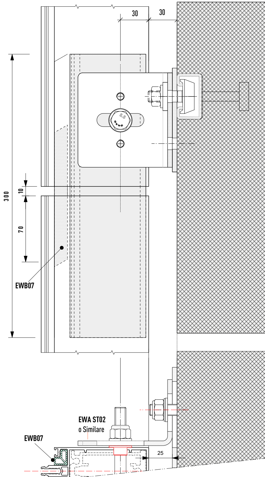
Canotto giunzione montanti L = 300 mm. Upright junction sleeve L = 300mm.
