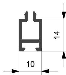
R 6229 Peso 0.673 kg./ml. -- mm. 550.0
